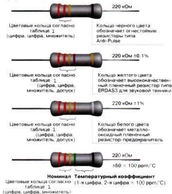
Рис. 4 Нестандартная цветовая маркировка.
